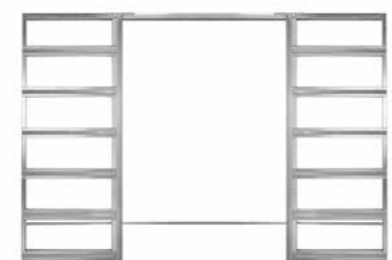
versione cartongesso
