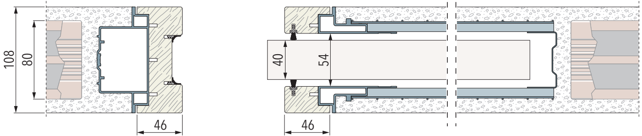
Parete Finita 125 mm - Tramezza 100 mm
