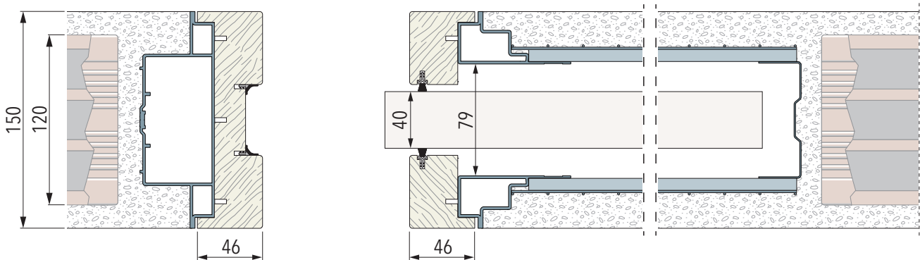
Parete Finita 150 mm - Tramezza 120 mm
