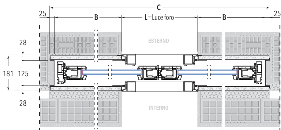
Esempio realizzativo con profili in PVC VEKA
